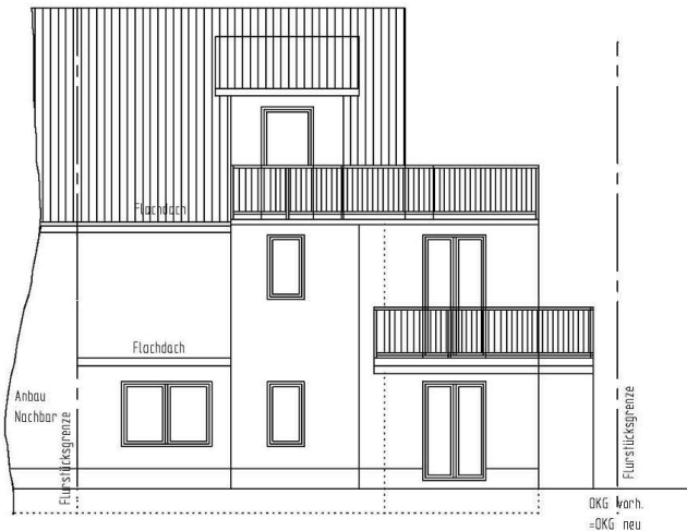
Ansicht West
