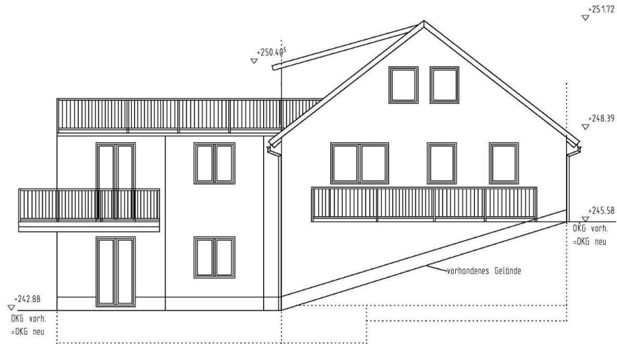
Ansicht Süd
