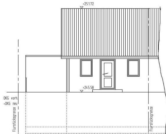
Ansicht Ost
